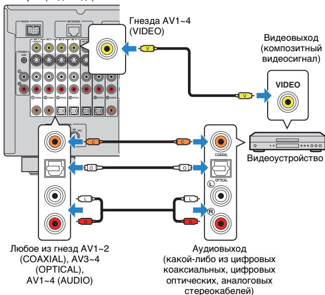
Аппарат (вид сзади)
