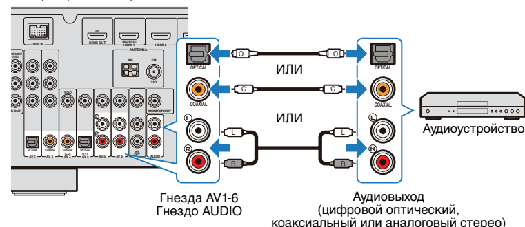
Аппарат (вид сзади)
